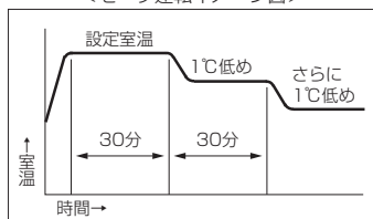
<セーブ運転イメージ図>
