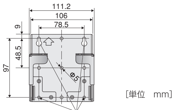
壁面取り付け穴（4カ所）
