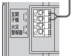
ドアホン親機(背面)
