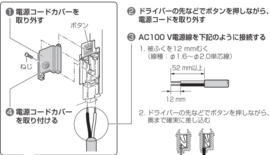
ドアホン親機(背面)
