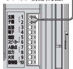
ドアホン親機(背面)
